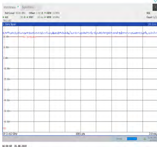
NTNV-11ax20MIMO-Ant7-2412
