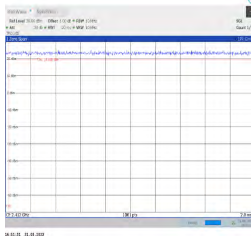
NTNV-11ax20MIMO-Ant9-2412
