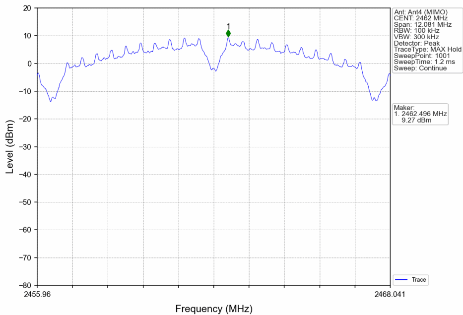
802.11b_HCH_2462MHz_Ant4 (MIMO)_NTNV
