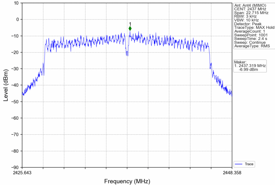
802.11ac(VHT20)_MCH_2437MHz_MIMO_NTNV
