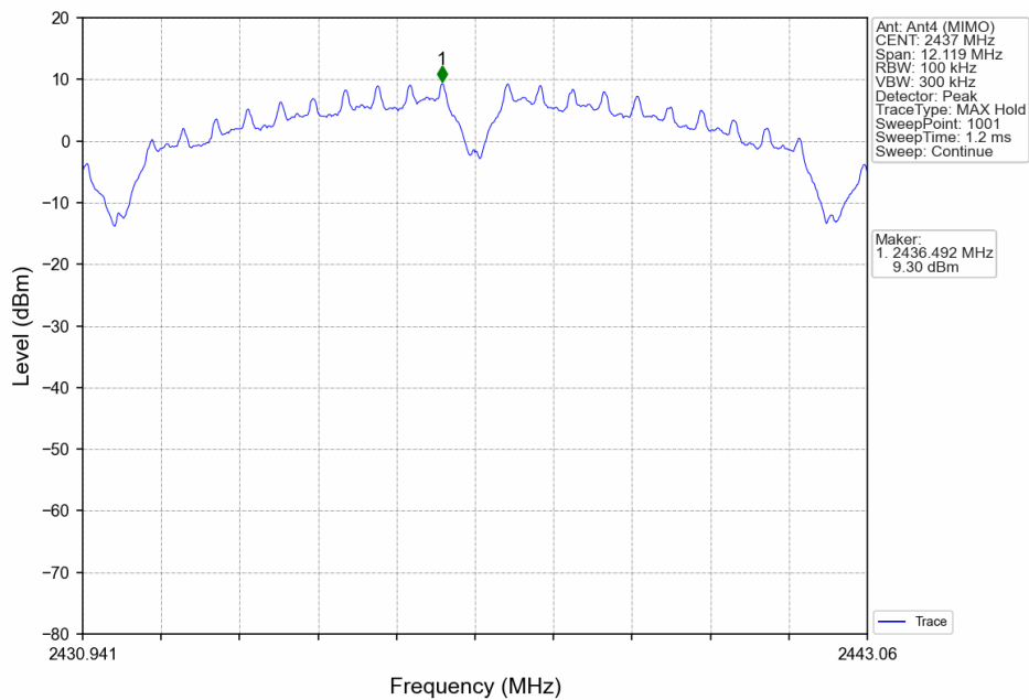
802.11b_MCH_2437MHz_Ant4 (MIMO)_NTNV
