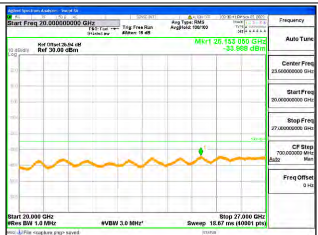
B38-20G-27G / 20MHz / High CH / QPSK
