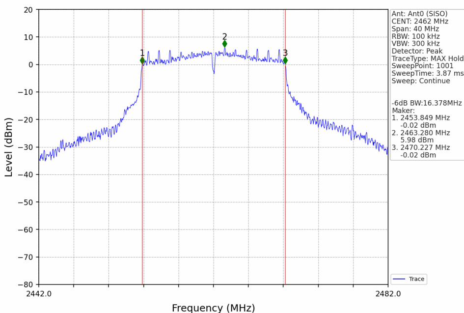
802.11g_HCH_2462MHz_Ant0 (SISO)_NTNV
