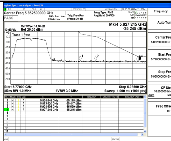
11N40MIMO-Ant1-5795-PASS
