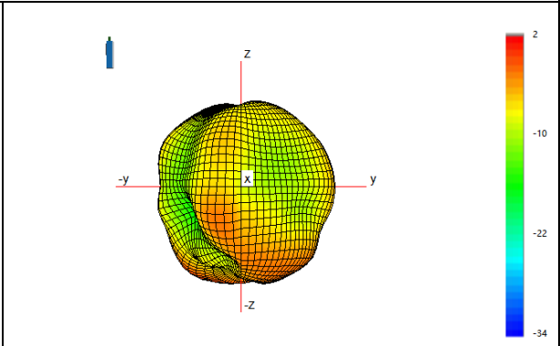
Ant7: 1575Mhz
