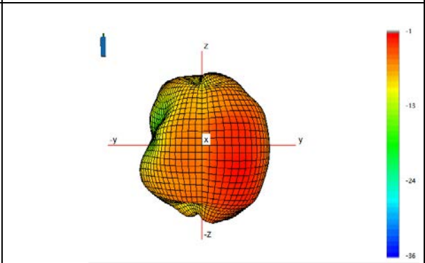
Ant7: 5500Mhz
