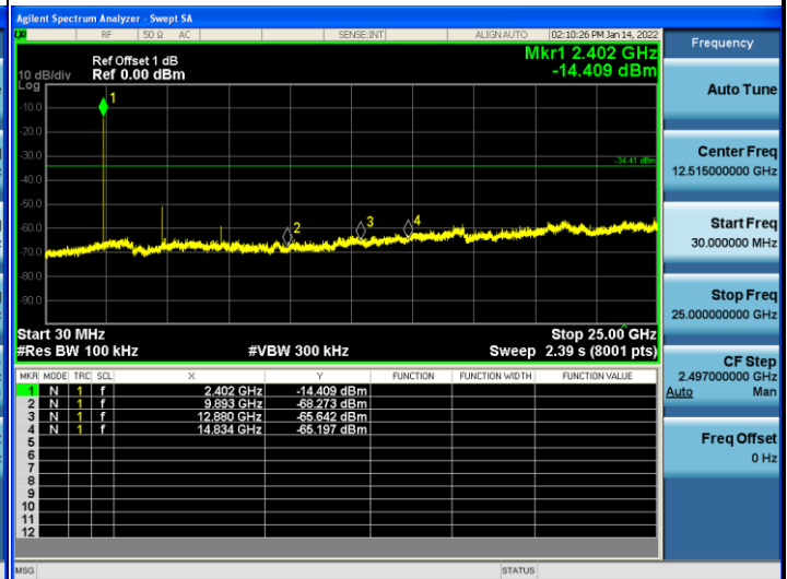
Mode 2 CH00(2402MHz)
