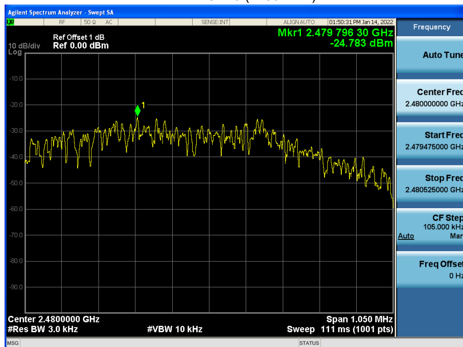
Mode 1 CH19 (2480 MHz)
