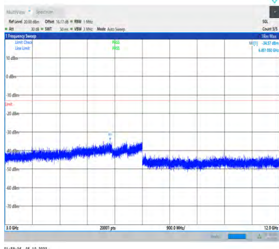
1-N66-PC3-15-40-L-1-DFT-QPSK-Inner_1RB_Left-1 @1-3000-12000-Ant1-6451.05--34.57--13-PASS
