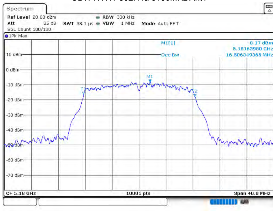
OBW NVNT 802.11a 5180MHz Ant1
