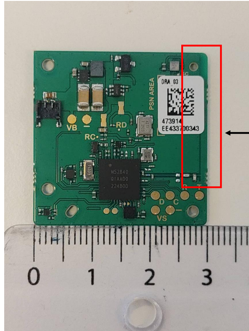
PCB bottom
