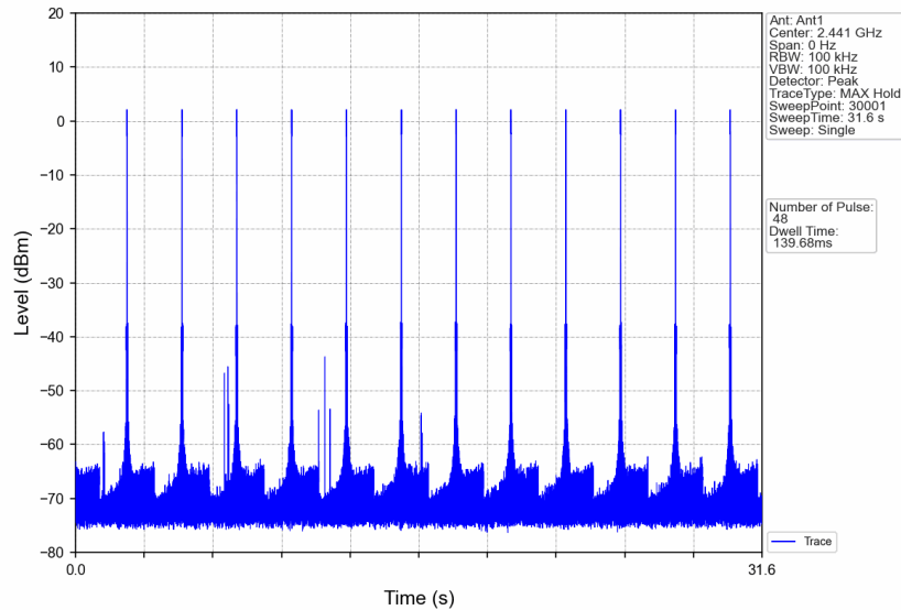
8DPSK_3DH1_HOPP_Ant1_NTNV
