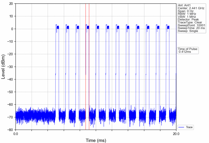
Pi/4DQPSK_2DH1_HOPP_Ant1_NTNV
