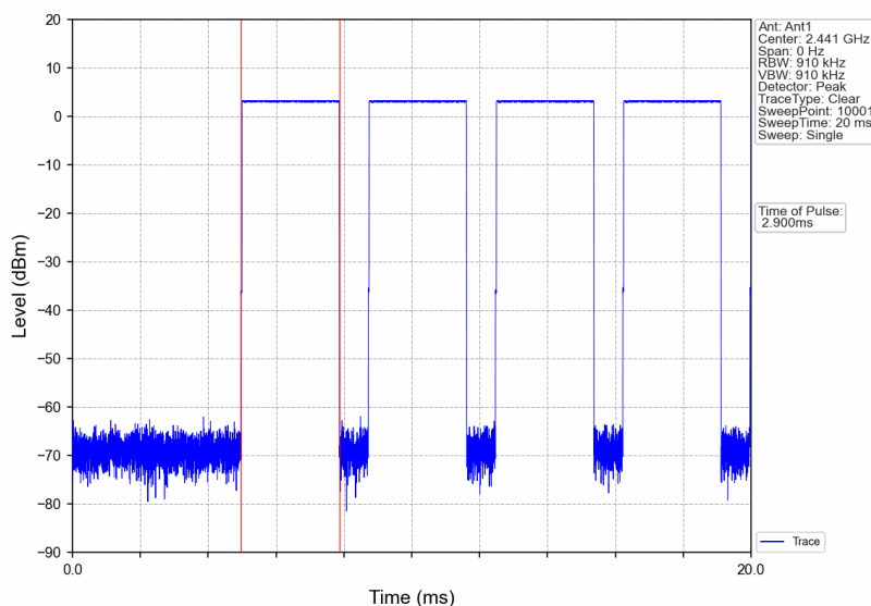
GFSK_DH5_HOPP_Ant1_NTNV
