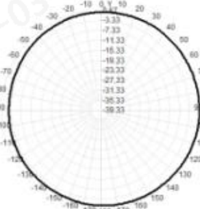
H 面
