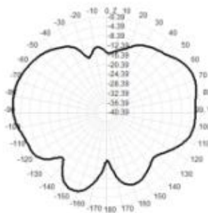
E 面
