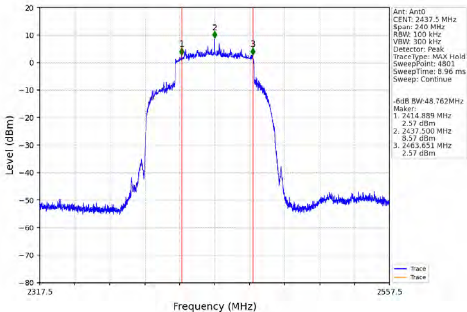
60M_MCH_2437.5MHz_Ant0_NTNV
