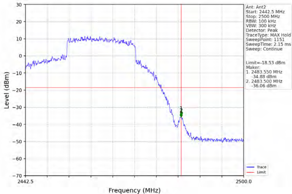
20M_HCH_2462.5MHz_Ant2_NTNV
