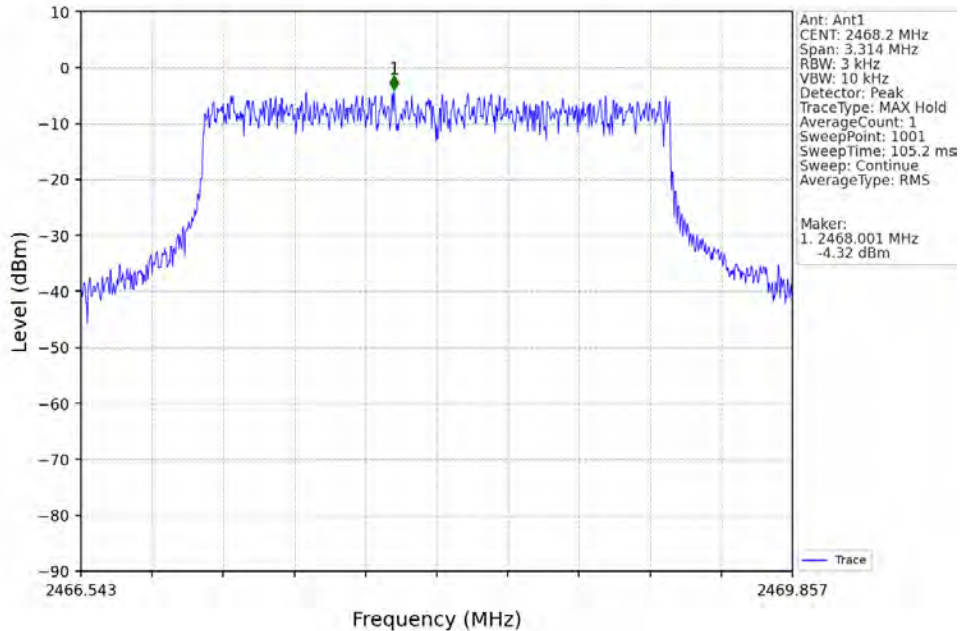
3M_HCH_2468.2MHz_MIMO_NTNV
