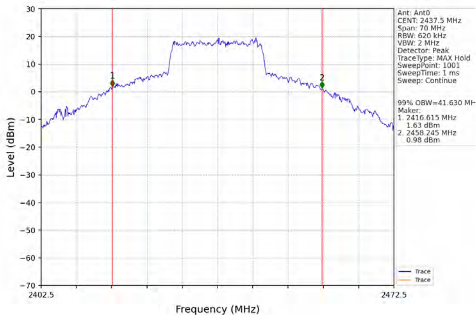
20M_MCH_2437.5MHz_Ant0_NTNV
