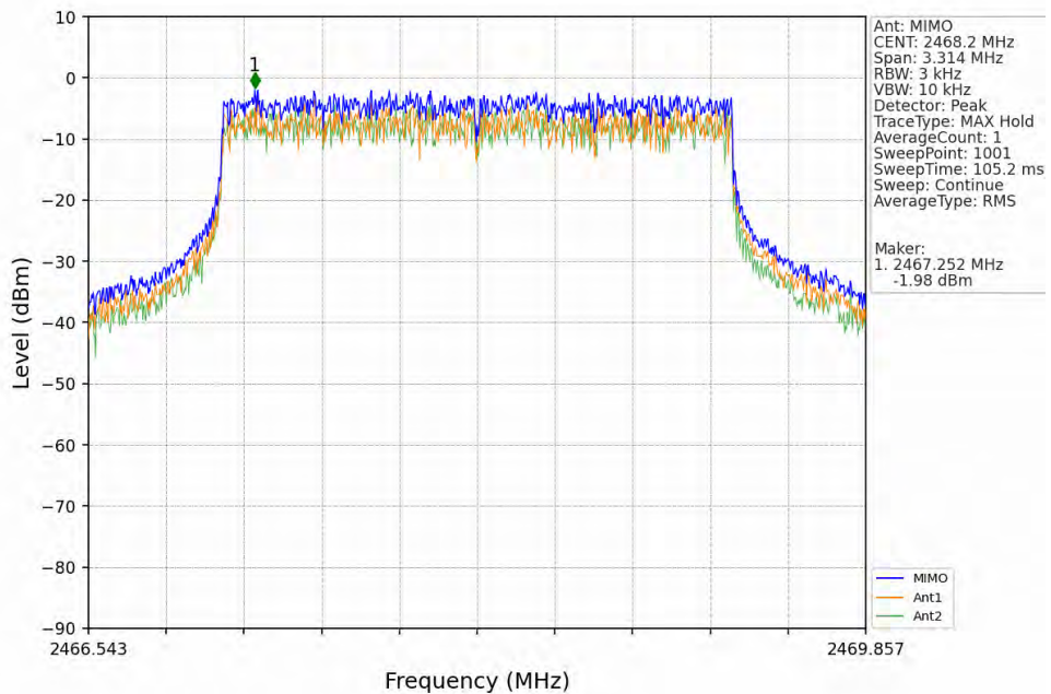
3M_HCH_2468.2MHz_MIMO_NTNV
