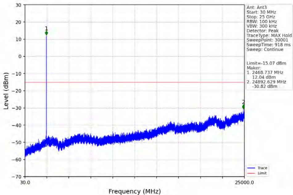
1.4M_HCH_2469.12MHz_Ant3_NTNV
