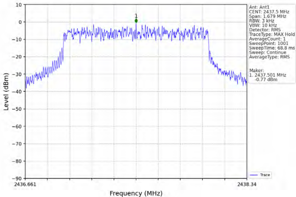
1.4M_MCH_2437.5MHz_MIMO_NTNV
