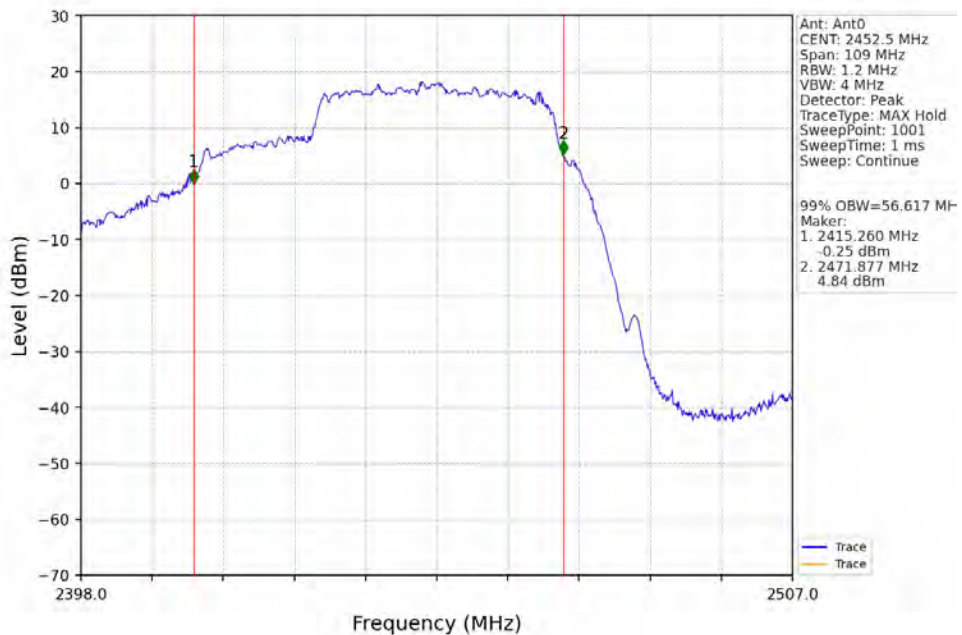
40M_HCH_2452.5MHz_Ant0_NTNV
