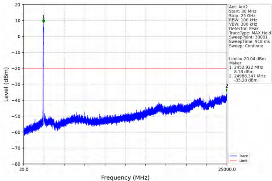
40M_HCH_2452.5MHz_Ant2_NTNV
