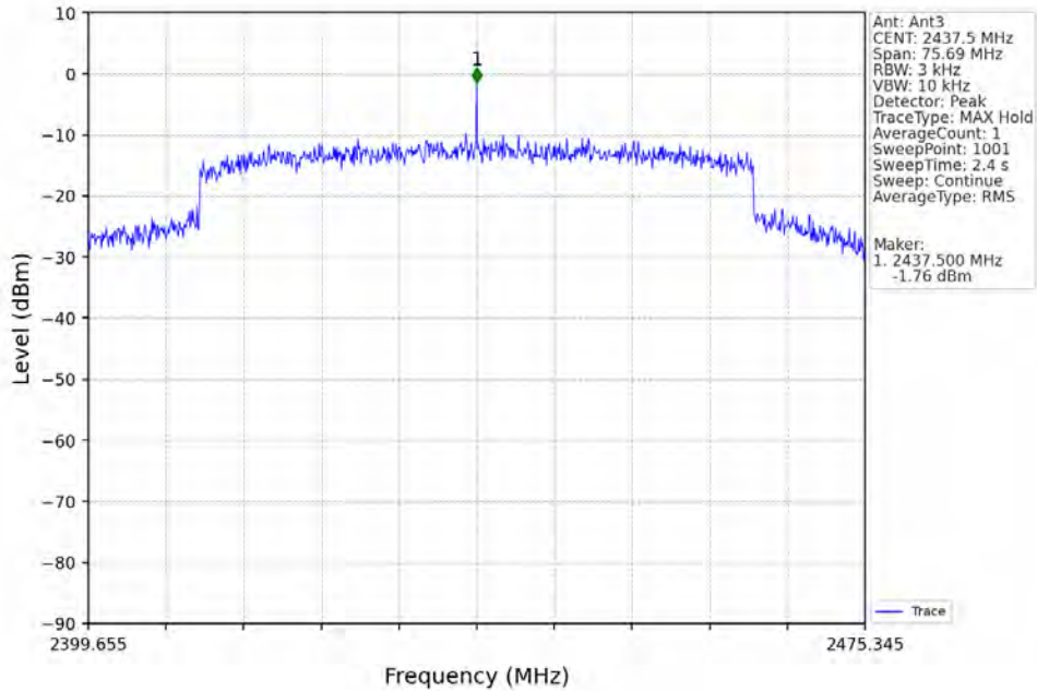
60M_MCH_2437.5MHz_MIMO_NTNV
