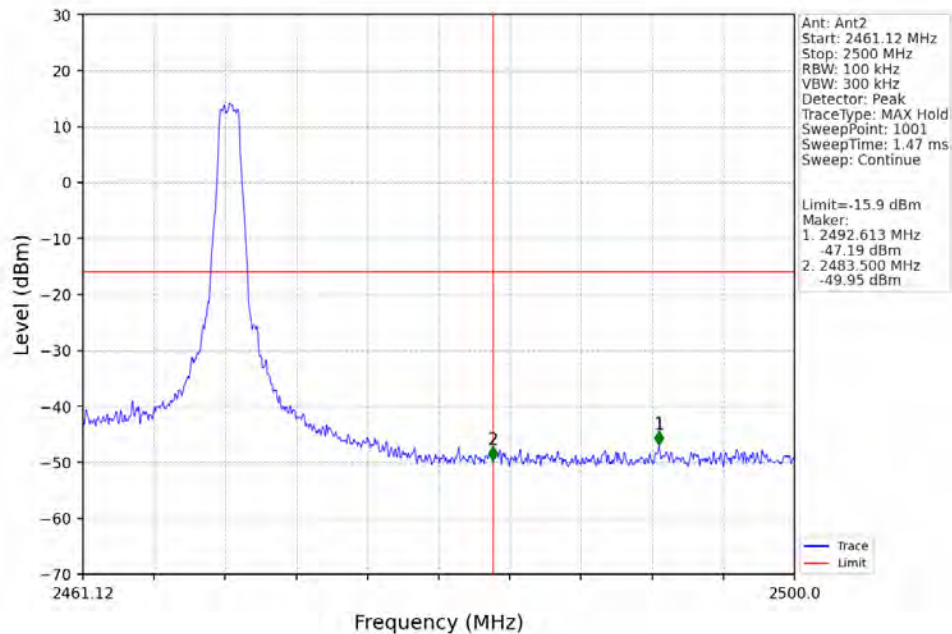
1.4M_HCH_2469.12MHz_Ant2_NTNV
