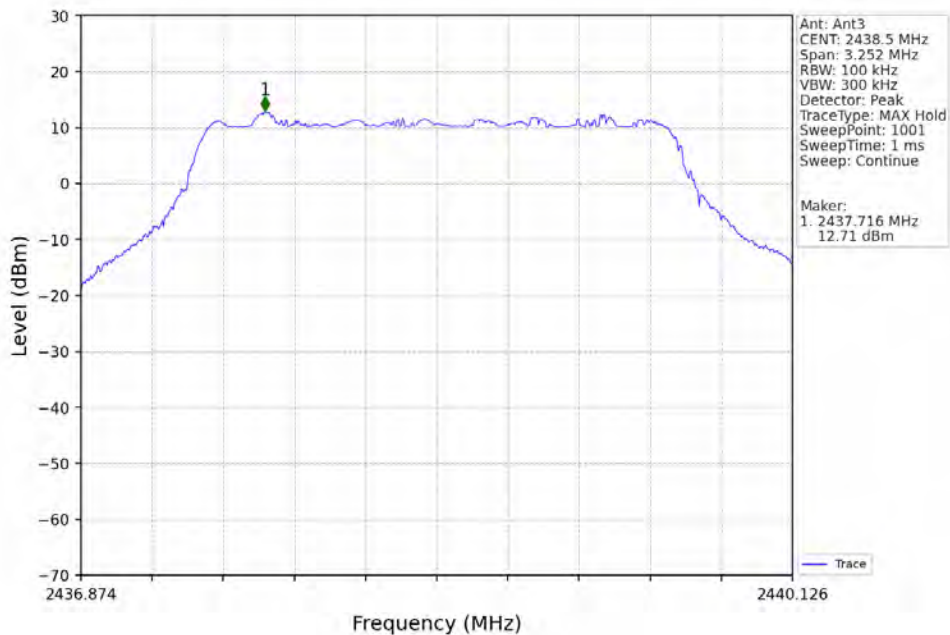
3M_MCH_2438.5MHz_Ant3_NTNV
