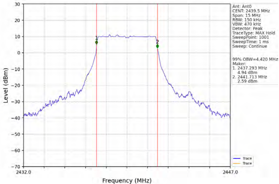
5M_MCH_2439.5MHz_Ant0_NTNV
