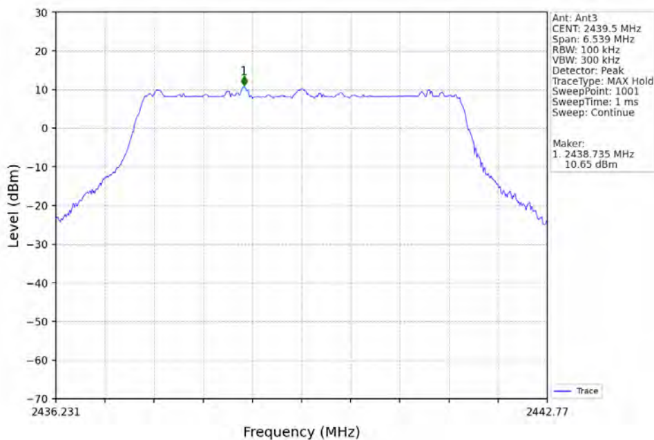
5M_MCH_2439.5MHz_Ant3_NTNV
