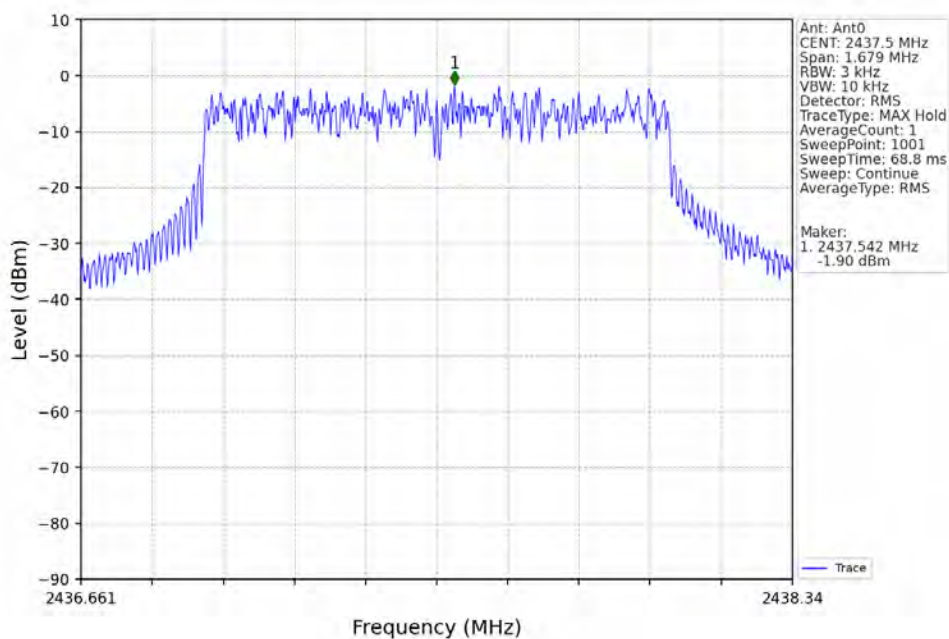
1.4M_MCH_2437.5MHz_Ant0_NTNV
