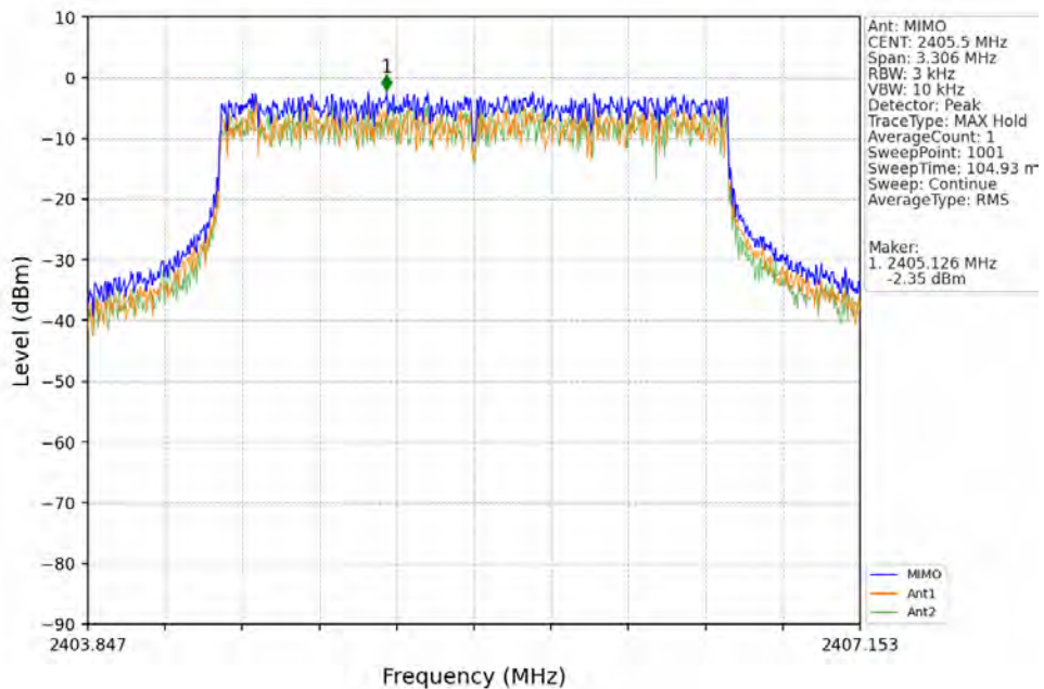
3M_LCH_2405.5MHz_MIMO_NTNV
