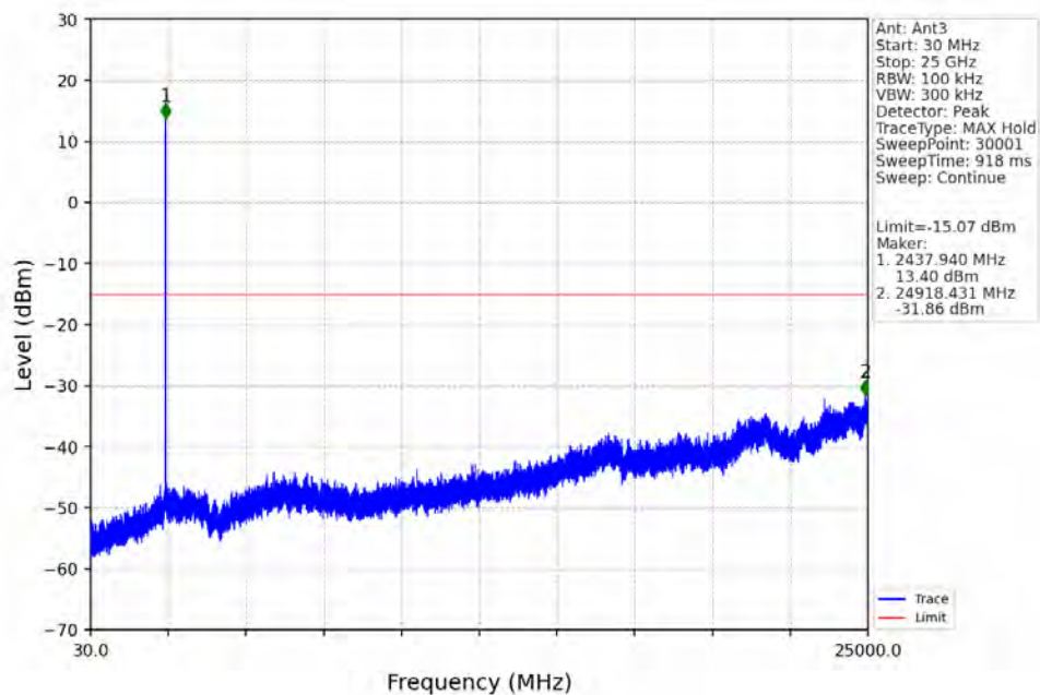
1.4M_MCH_2437.5MHz_Ant3_NTNV
