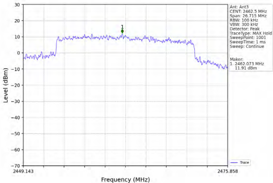
20M_HCH_2462.5MHz_Ant3_NTNV
