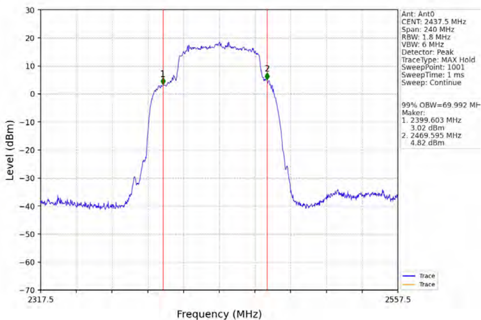
60M_MCH_2437.5MHz_Ant0_NTNV
