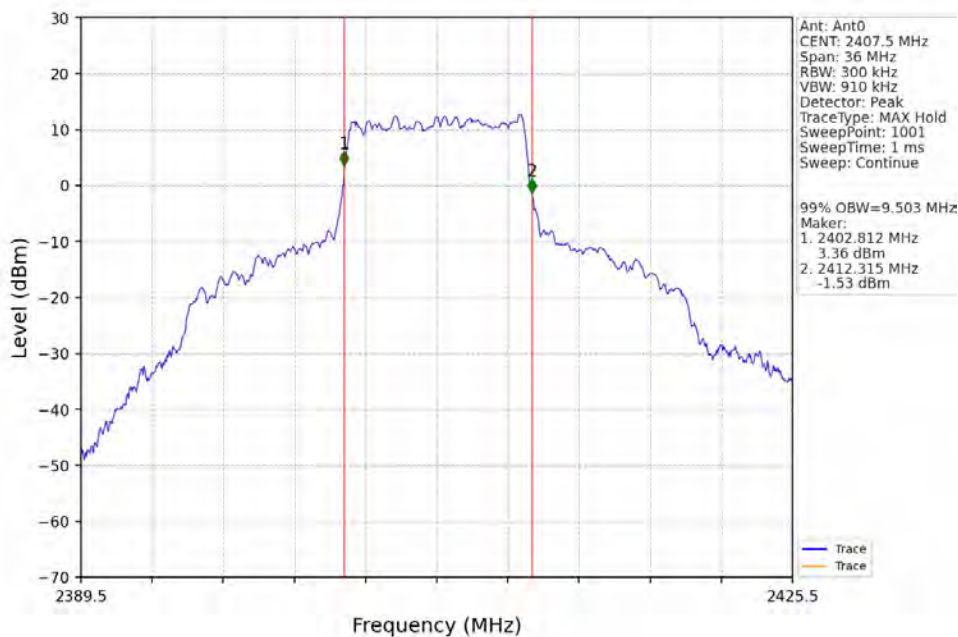
10M_LCH_2407.5MHz_Ant0_NTNV
