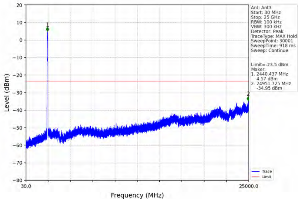
60M_MCH_2437.5MHz_Ant3_NTNV
