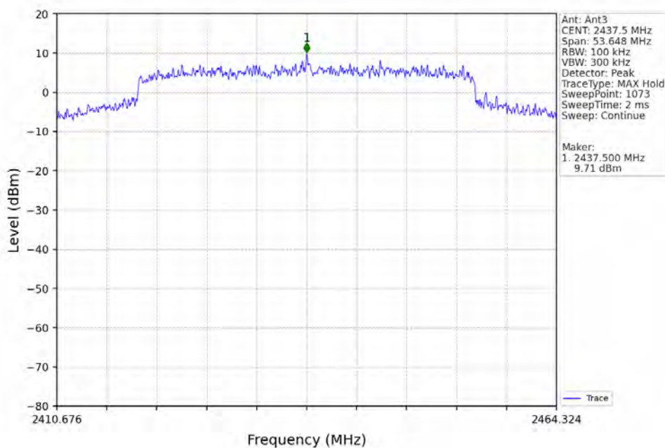
40M_MCH_2437.5MHz_Ant3_NTNV
