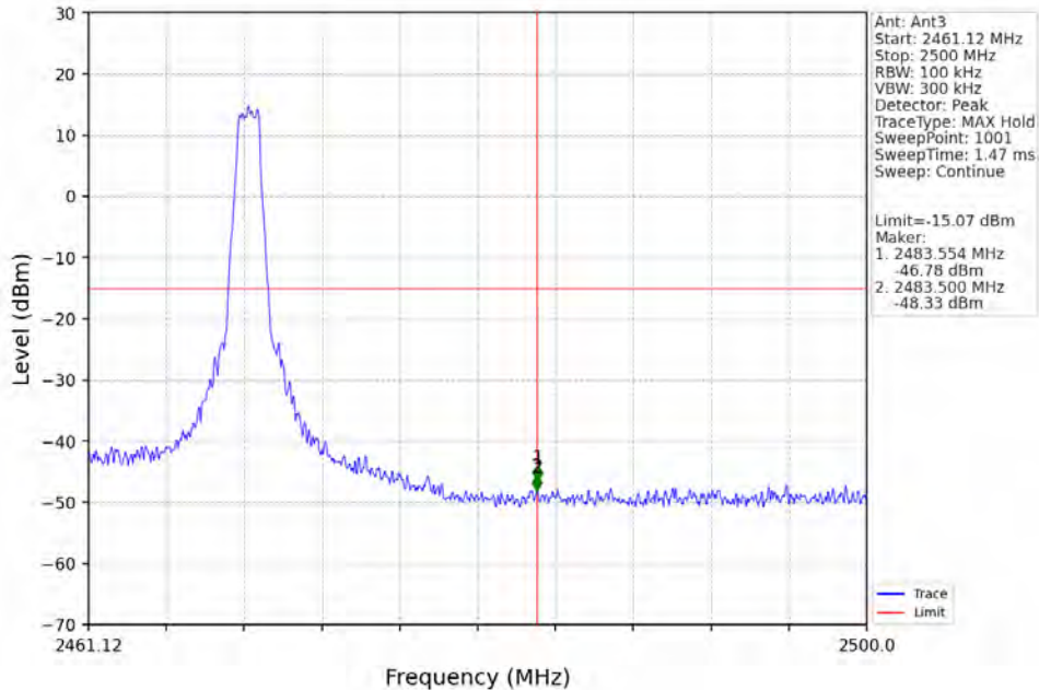
1.4M_HCH_2469.12MHz_Ant3_NTNV
