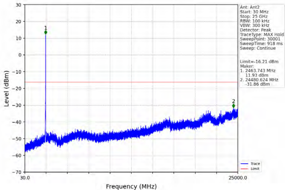
10M_HCH_2467.5MHz_Ant2_NTNV
