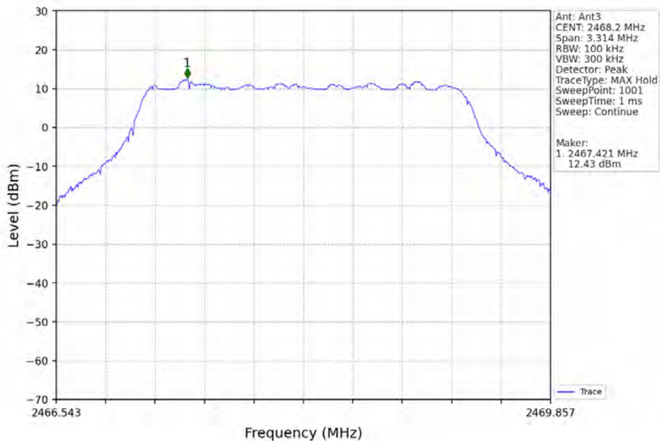
3M_HCH_2468.2MHz_Ant3_NTNV
