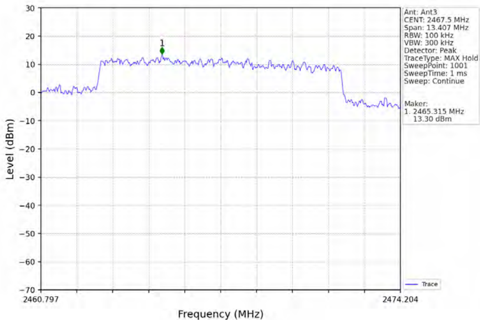
10M_HCH_2467.5MHz_Ant3_NTNV
