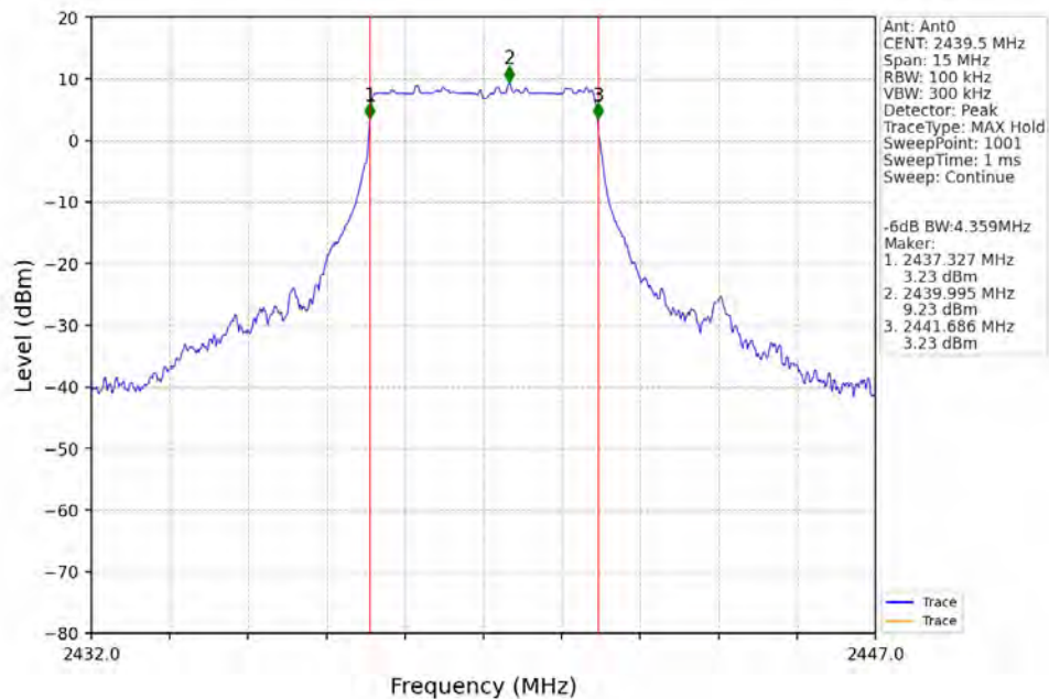
5M_MCH_2439.5MHz_Ant0_NTNV
