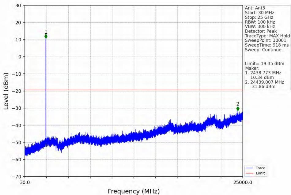
5M_MCH_2439.5MHz_Ant3_NTNV
