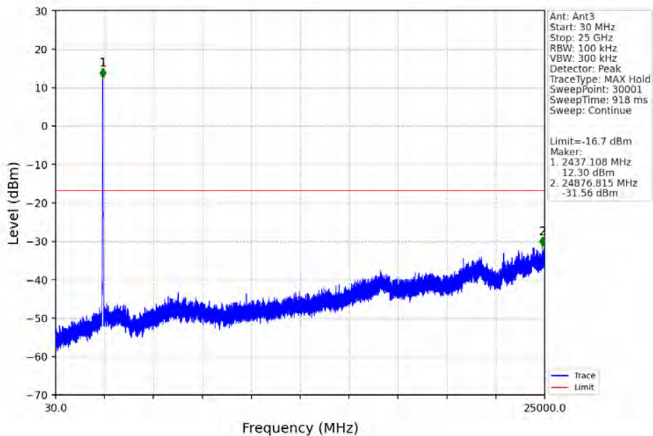
10M_MCH_2437.5MHz_Ant3_NTNV
