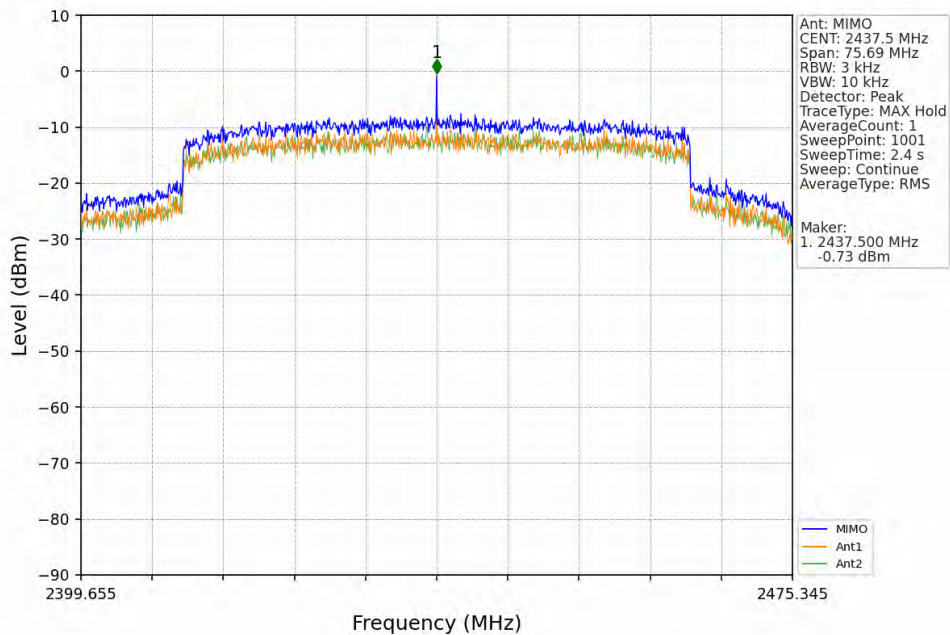
60M_MCH_2437.5MHz_MIMO_NTNV
