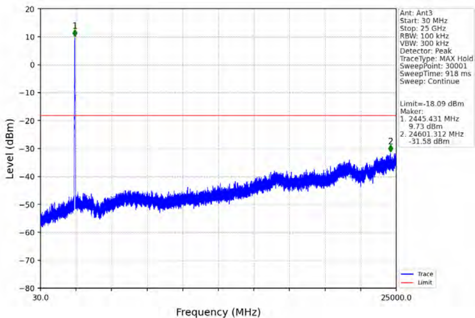
20M_MCH_2437.5MHz_Ant3_NTNV
