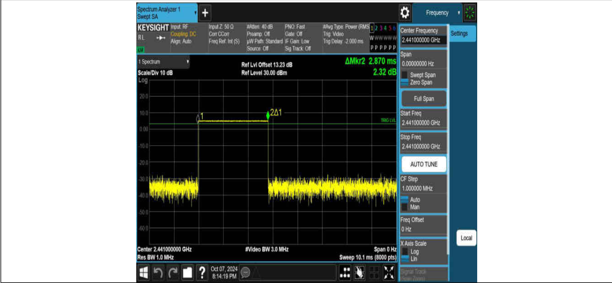
DH5_Ant1_Hop
