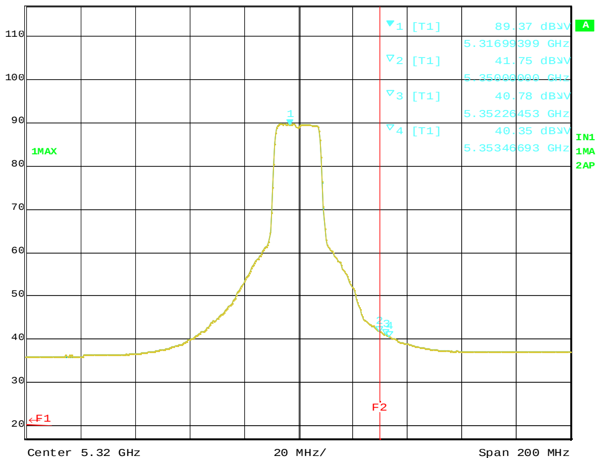
Plot 7-4 5320MHz TX mode (Average). R50 series
