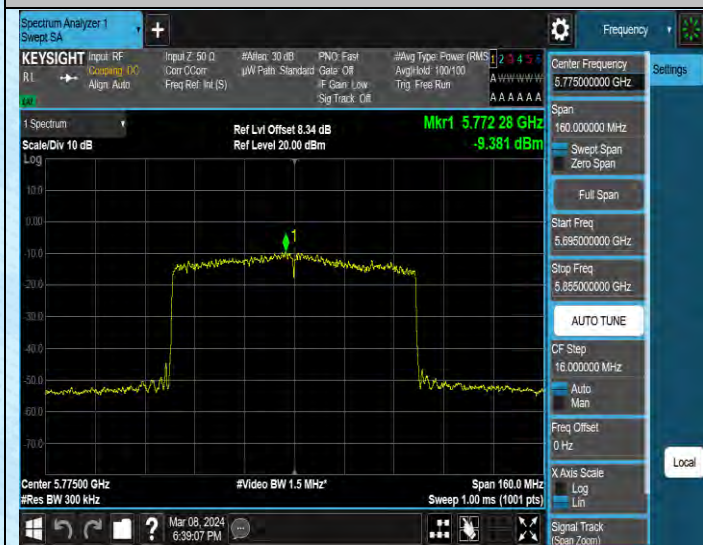
11AX80SISO-Ant1-5775-PASS
