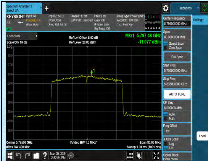
11AX40MIMO-Ant1-5795-PASS
