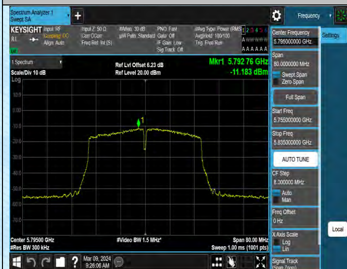
11N40MIMO-Ant1-5795-PASS
