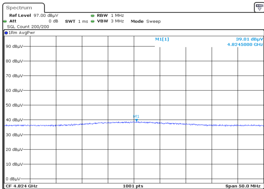
F1 X2 4824.0 Harmonic Vertical AVG
