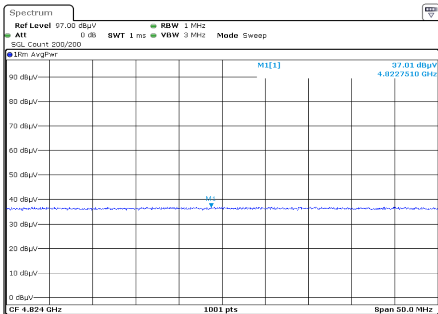
F1 X2 4824.0 Harmonic Horizontal AVG
