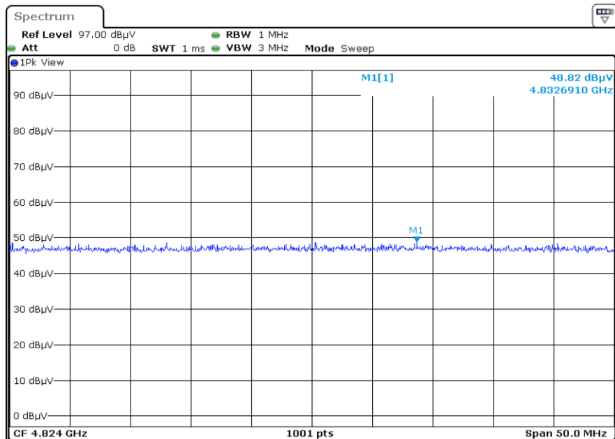
F1 X2 4824.0 Harmonic Horizontal PEAK
