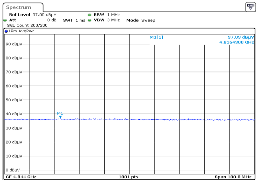
F1 X2 4844.0 Harmonic Horizontal AVG
