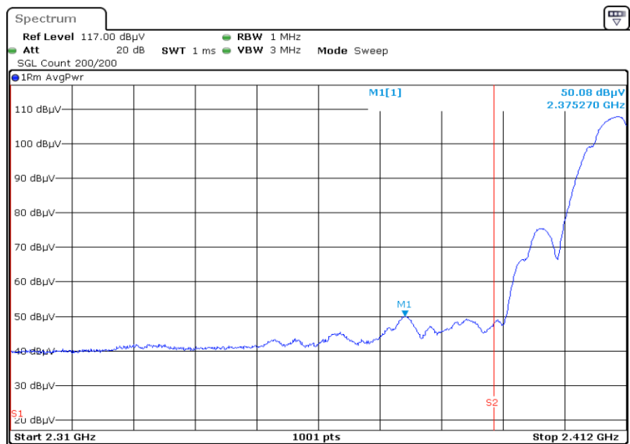
2412.0 F1 RestrictedBand Vertical AVG
