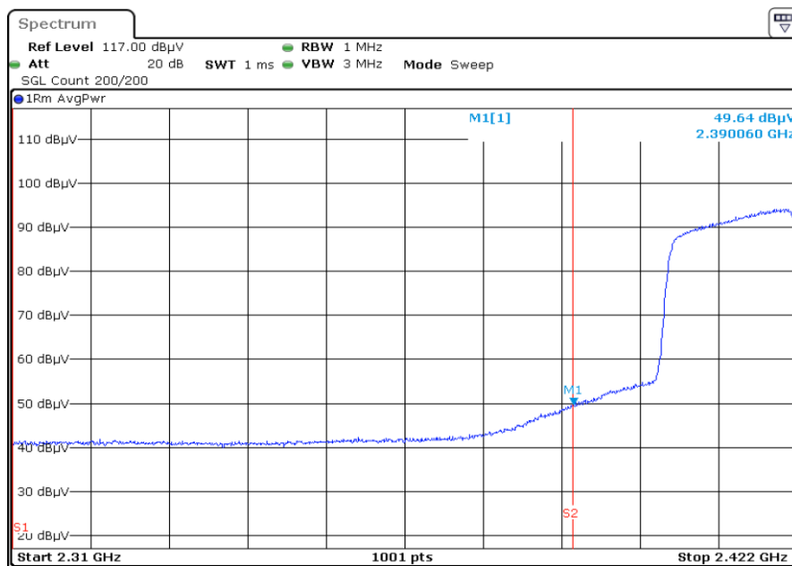
2422.0 F1 RestrictedBand Vertical AVG
