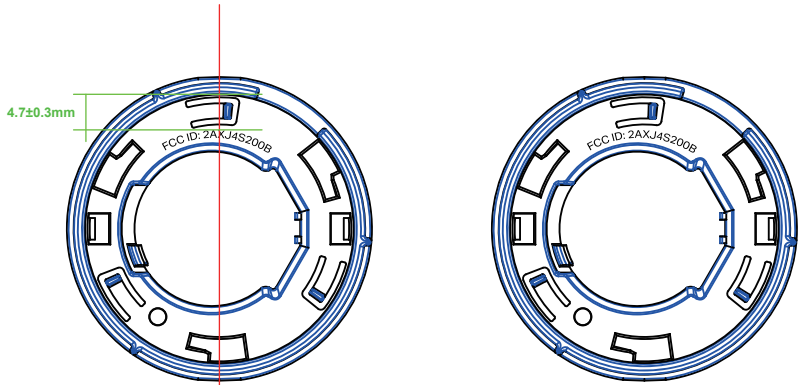
尺寸图
