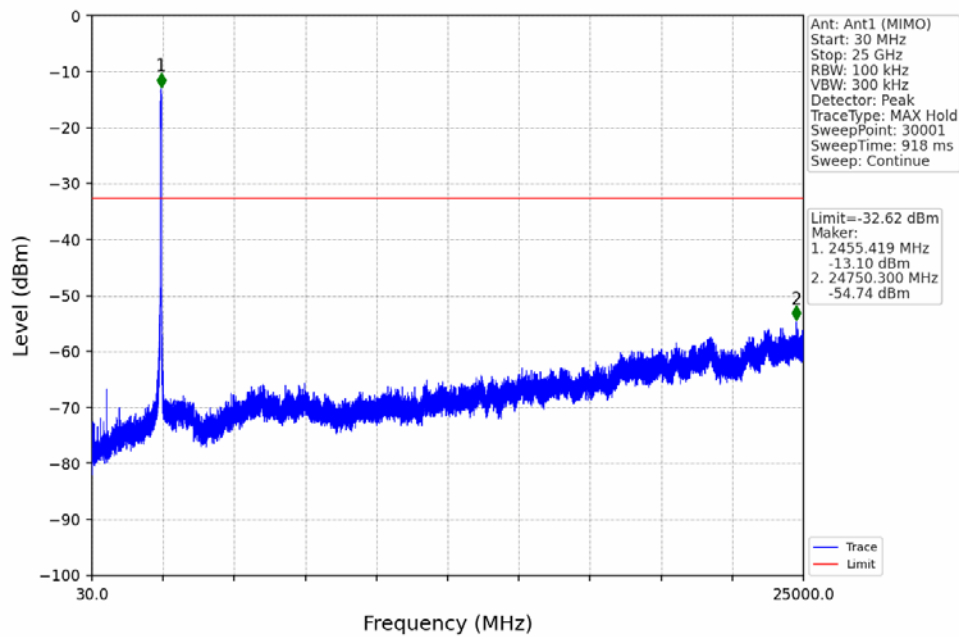
802.11ax(HEW40) HCH 2452MHz RU484 Left Ant1 (MIMO) NTNW
