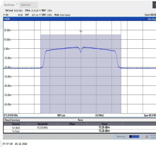
11AC40MIMO-Ant1-5310-TPC L-----14.69-87.80-0.57
