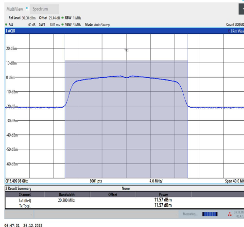
11AC20MIMO-Ant1-5500-TPC L-----11.20-91.89-0.37
