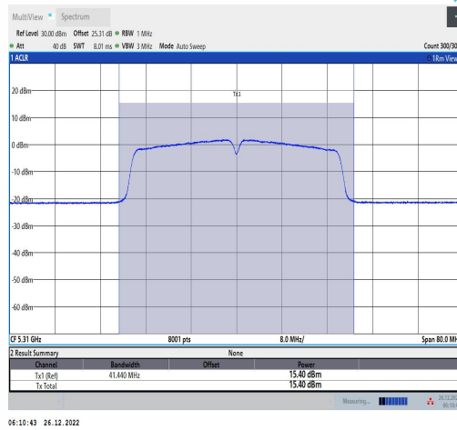
11N40MIMO-Ant1-5310-TPC L-----15.08-92.86-0.32
