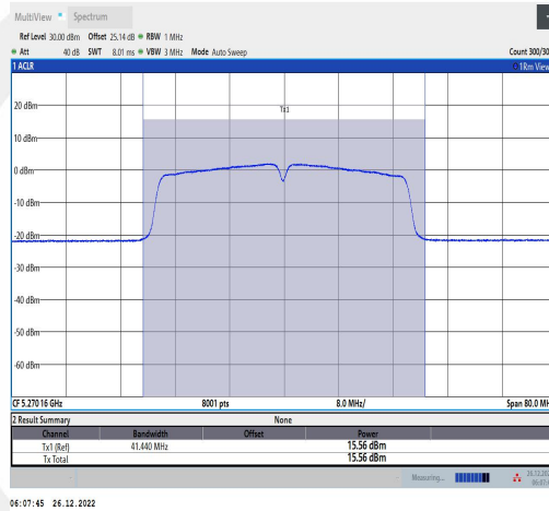
11N40MIMO-Ant1-5270-TPC L-----15.24-92.86-0.32
