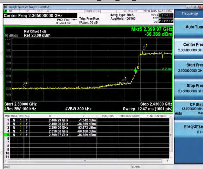
11AX40SISO_Ant2_Low_2422
