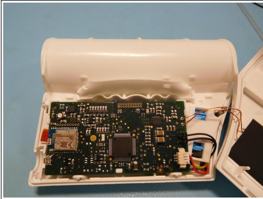
PCB TOP
