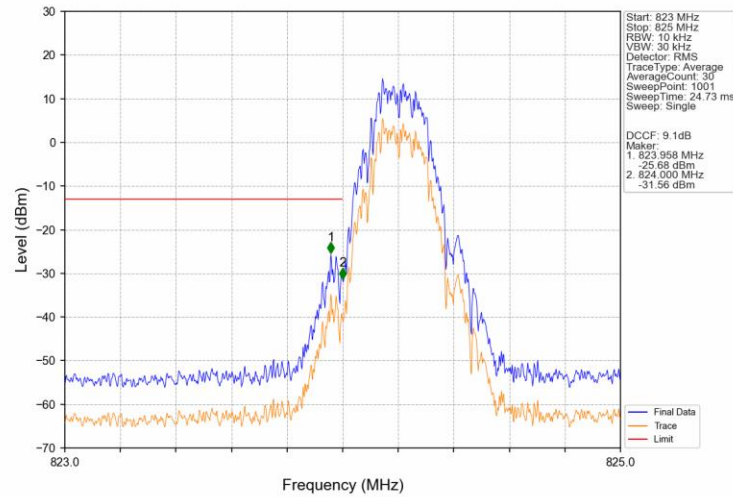
GSM850 GSM LCH 824.2MHz GSM NTN
