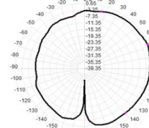
2480.0MHz Total(E2-YZ), Max: -0.14dB
