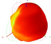
2500.0MHz H+V, ER: 40.6%
