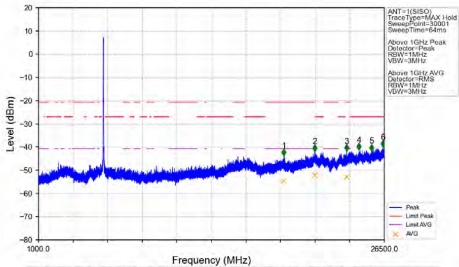
802.11a_MCH_5785MHz_Ant1_NTNV
