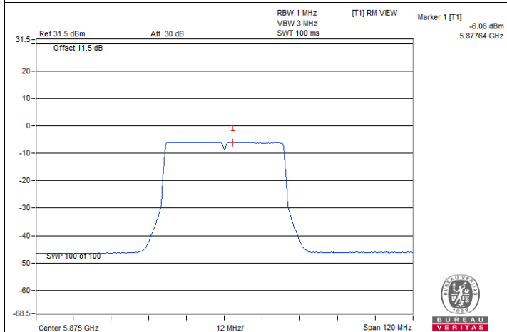
802.11be (EHT40) / Chain 1 : CH 175
