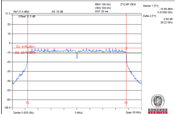
802.11be (EHT40) / Chain 0 : CH 167
