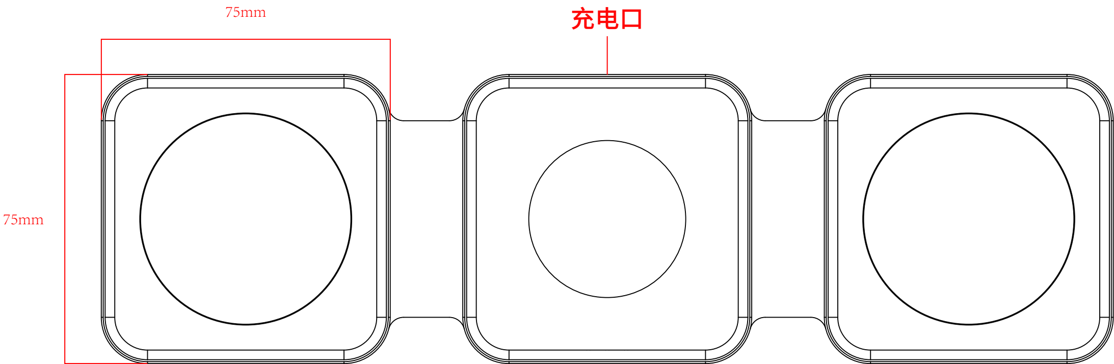
前面丝印 (A面)
