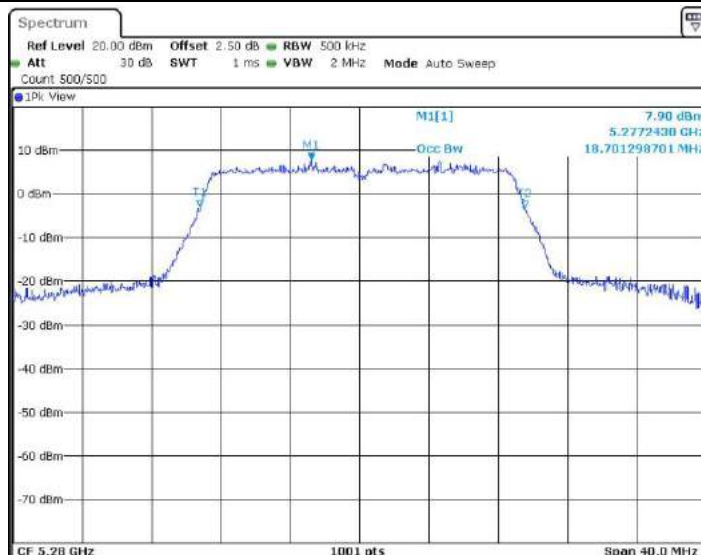
11N20SISO_Ant2_5280
