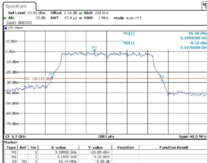
11N20MIMO_Ant1_5200
