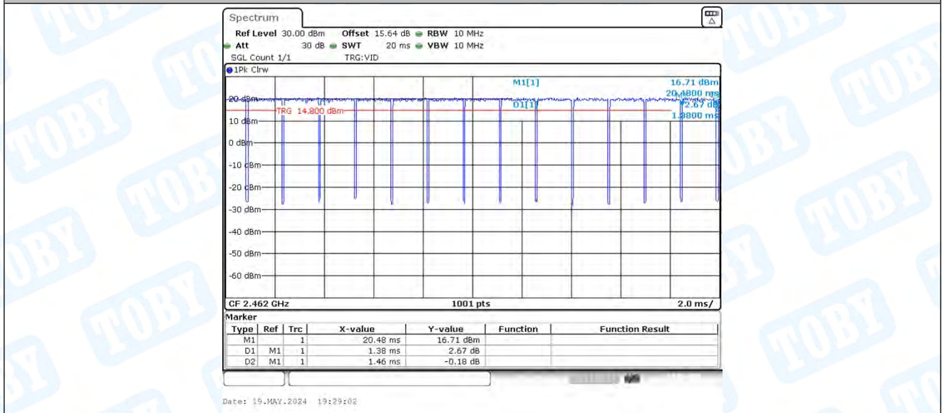
11G_Ant2_2462
