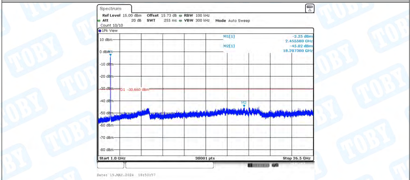
11N40MIMO_Ant2_2452_1000~26500
