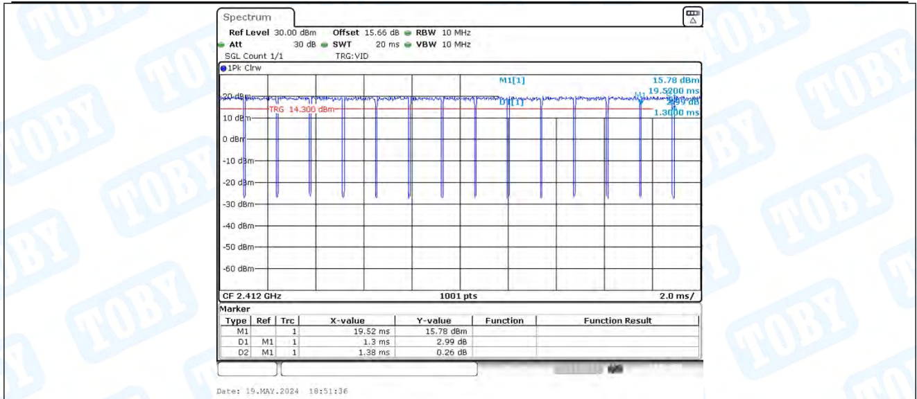
11N20MIMO_Ant2_2412
