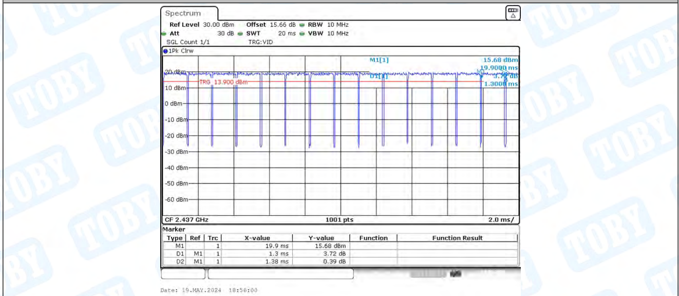
11N20MIMO_Ant2_2437
