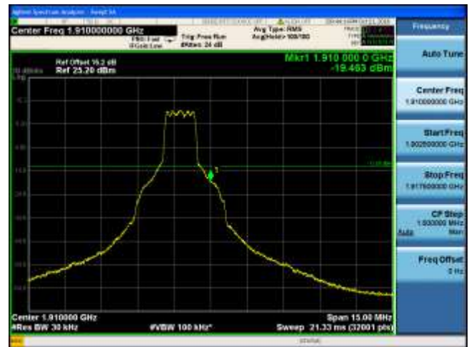
WCDMA Band II-CH9538
