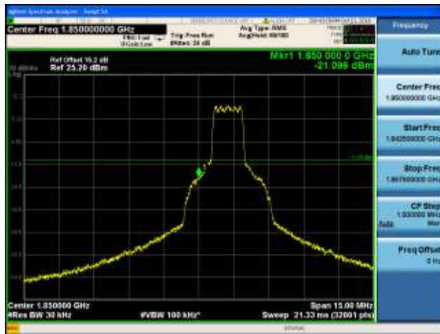
WCDMA Band II-CH9262
