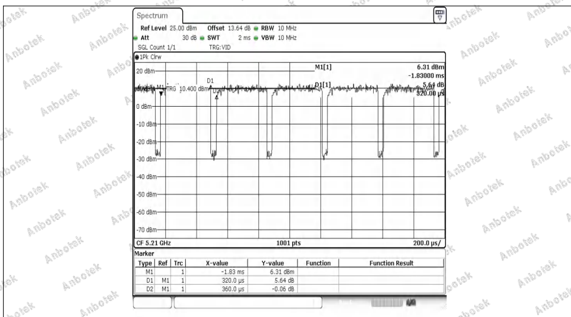
NTNV-11AC80SISO-Ant1-5210
