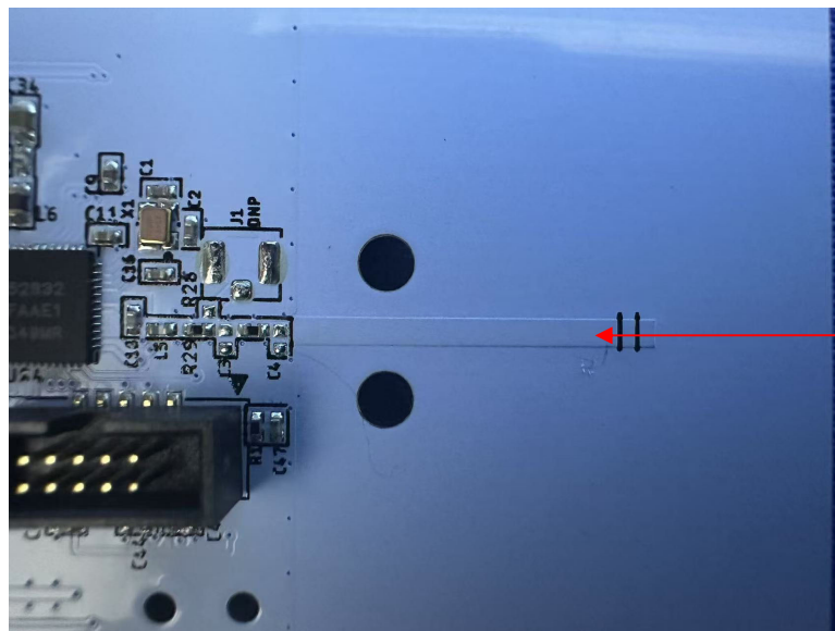
BLE Antenna
