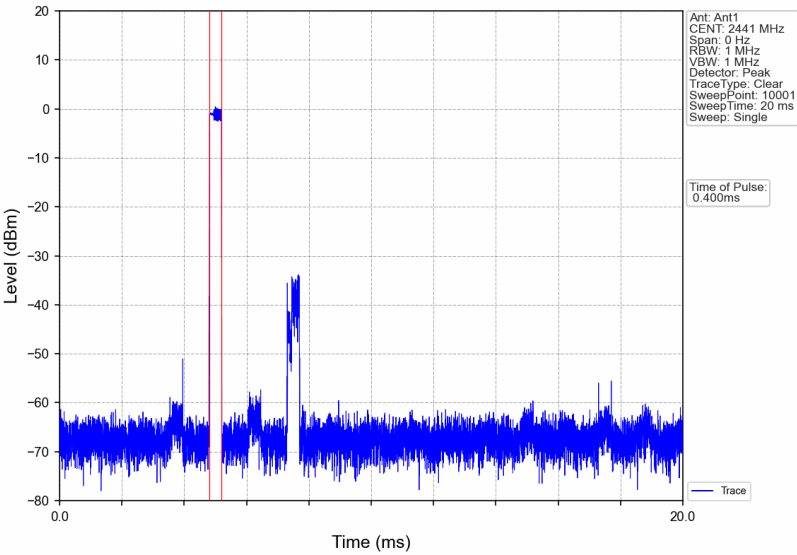
Pi/4DQPSK_2DH1_HOPP_Ant1_NTNV
