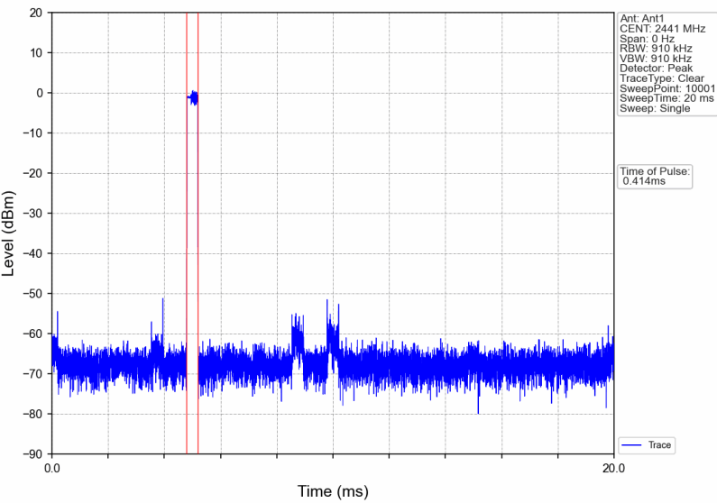
8DPSK_3DH1_HOPP_Ant1_NTNV
