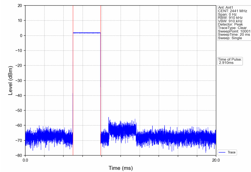
GFSK_DH5_HOPP_Ant1_NTNV
