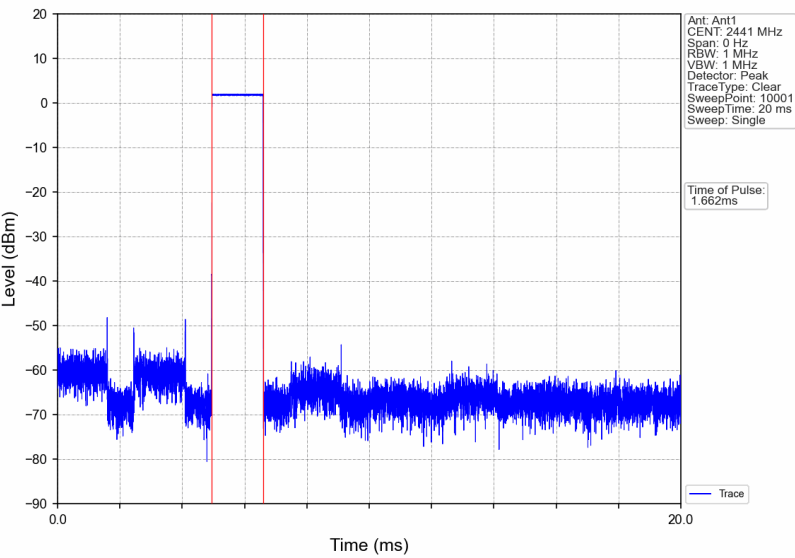
GFSK_DH3_HOPP_Ant1_NTNV
