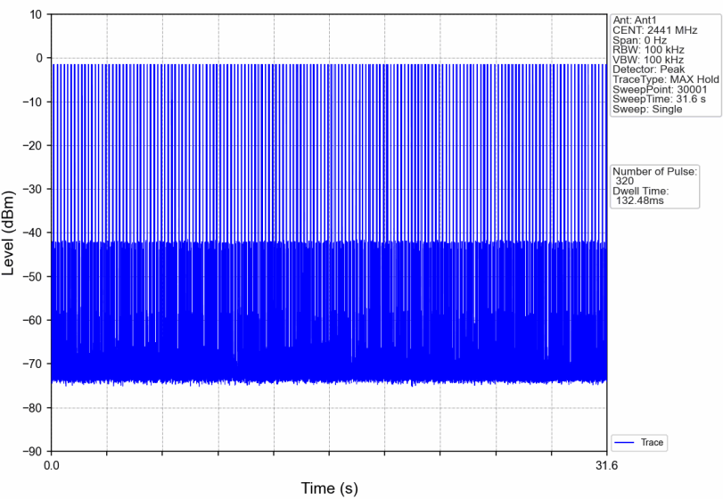
8DPSK_3DH1_HOPP_Ant1_NTNV
