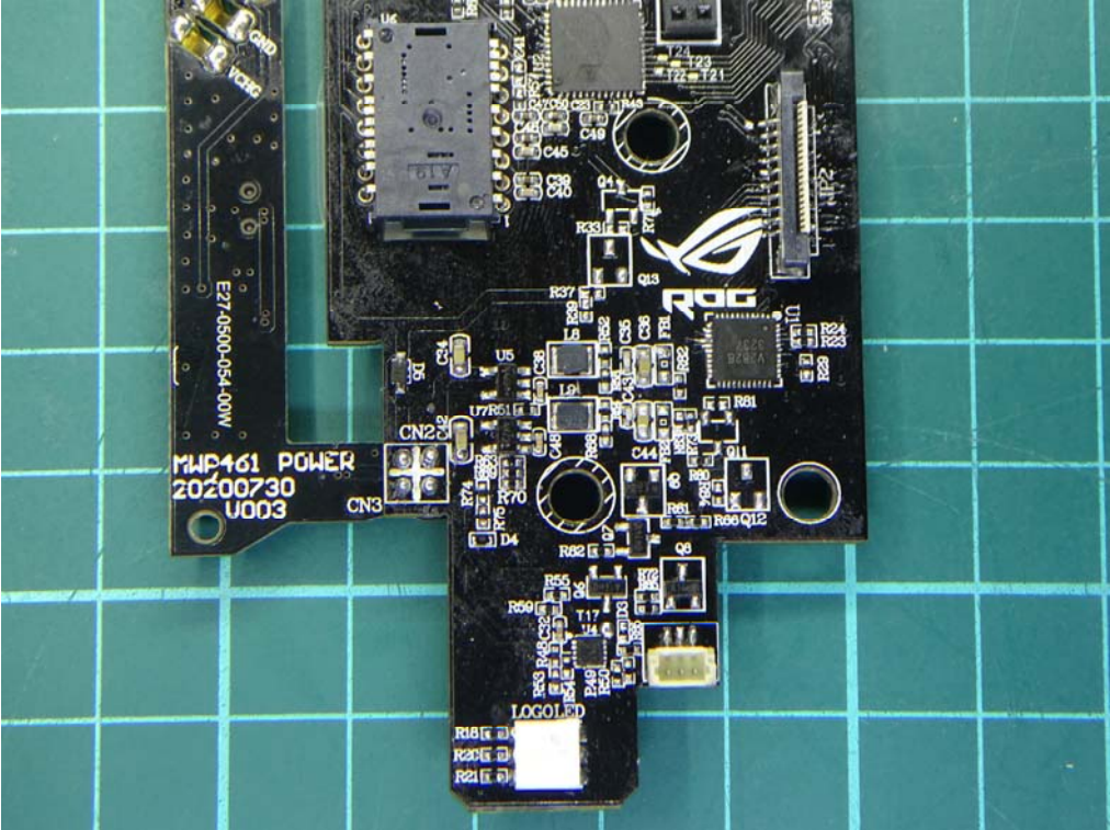
(24) EUT Photo
