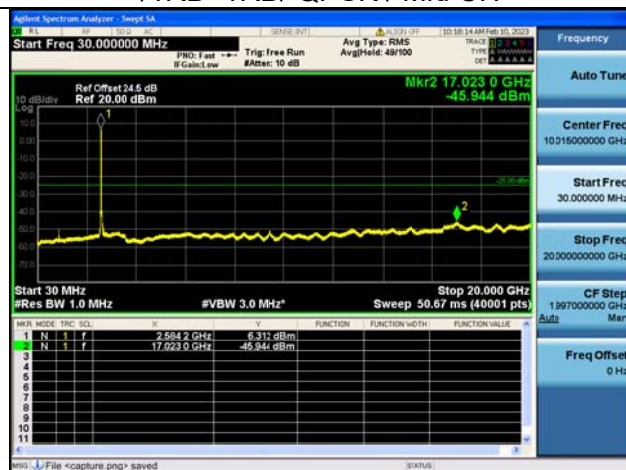
Band41C-30M-20G / 15MHz+15MHz /75RB+75RB/ QPSK / Mid CH
