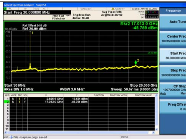
Band41C-30M-20G / 20MHz+10MHz /1RB+1RB/ QPSK / Mid CH
