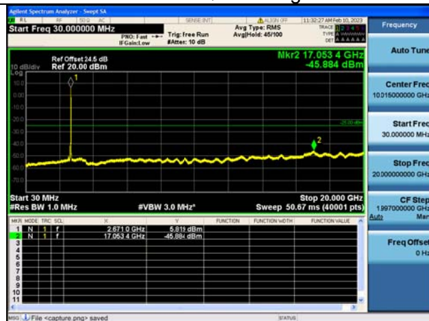
Band41C-30M-20G / 10MHz+15MHz /50RB+75RB/ QPSK / High CH
