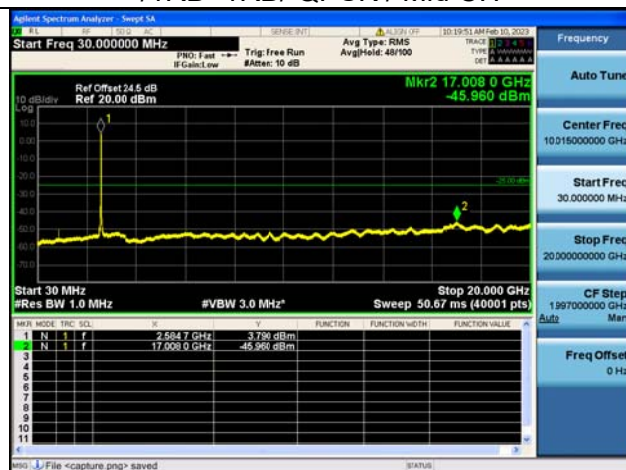
Band41C-30M-20G / 15MHz+20MHz /75RB+100RB/ QPSK / Mid CH
