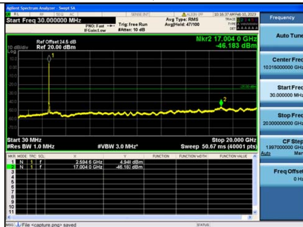
Band41C-30M-20G / 20MHz+10MHz /100RB+50RB/ QPSK / Mid CH
