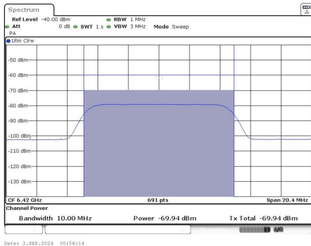
802.11be (BE320) / 6420MHz (Upper edge) Threshold Level (TL) = -69.94 dBm
