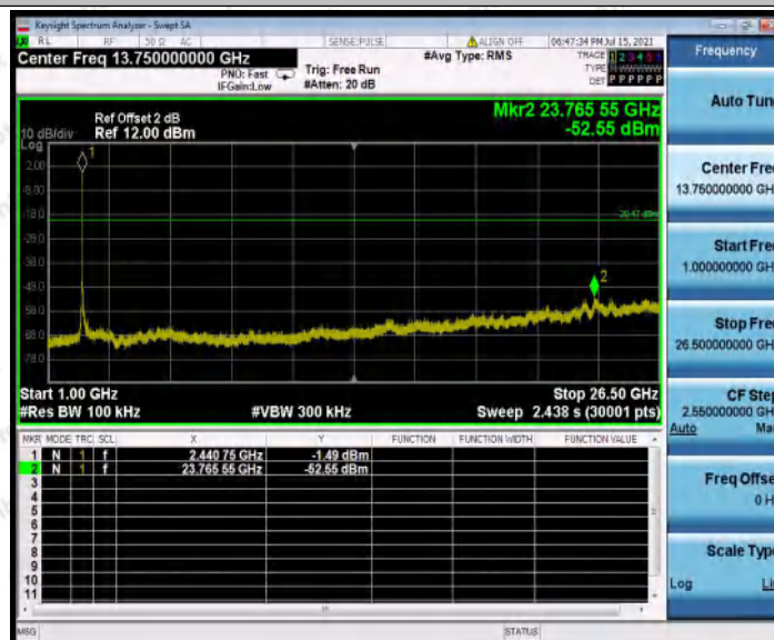
11N20_Ant1_2437_1000~26500
