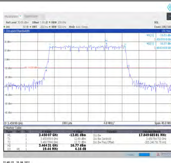
1-N78-3450-3550--30-20-L-2-DFT-PI2BPSK-Outer_Full -50@0-Ant1-17.85-19.440-≤20-PASS
