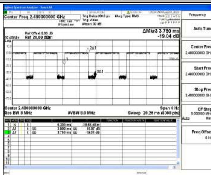
2D41_Ant1_2480
