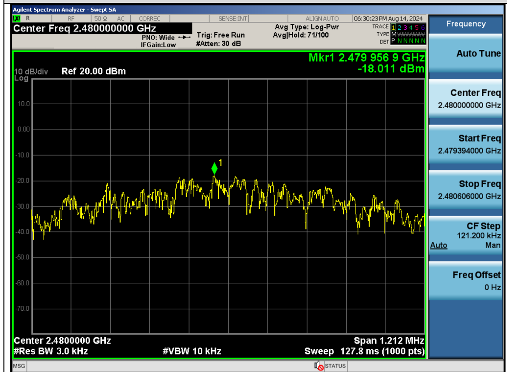
Test_Graph_2.4G_ANT1_2480_PSD
