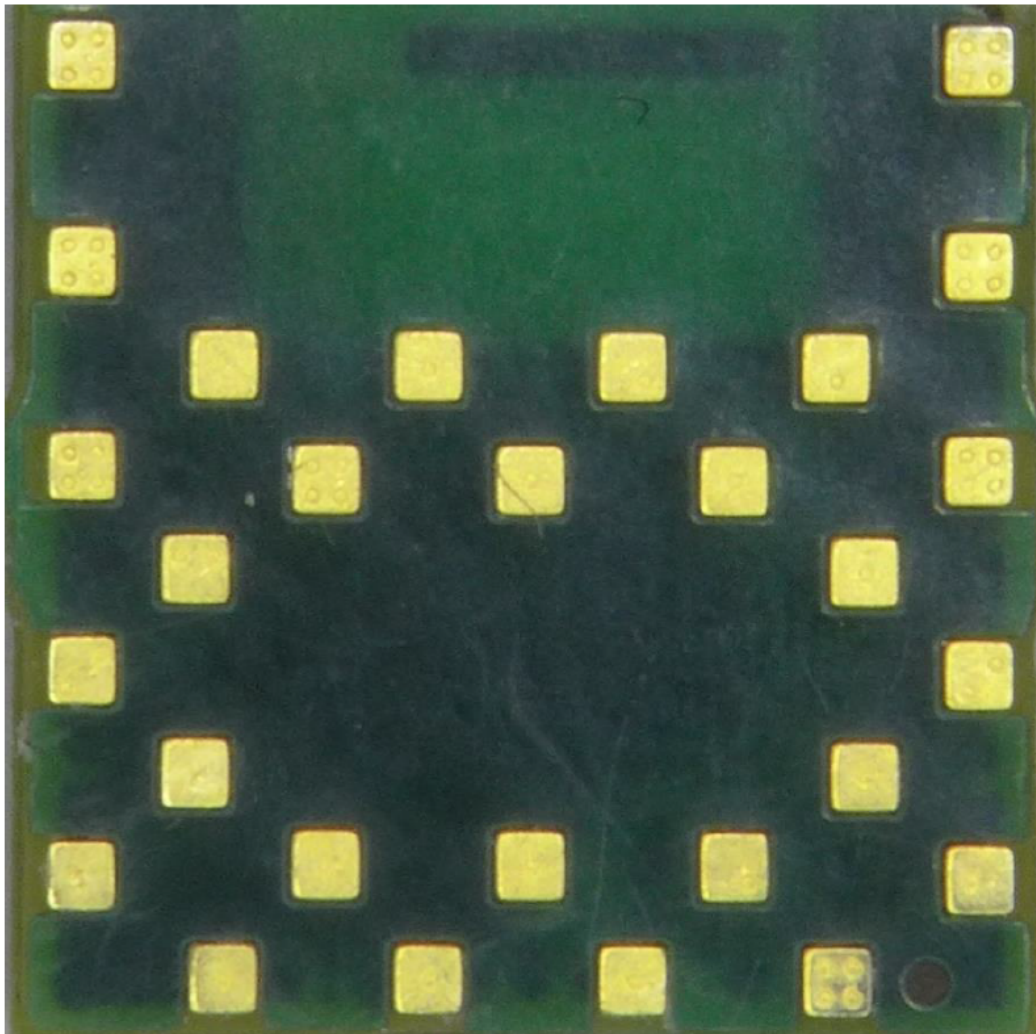
EUT PAN1326C2 back side
