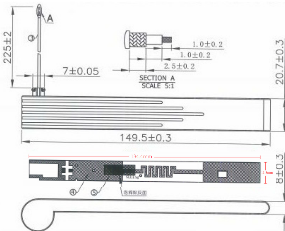
2.4G Antenna
