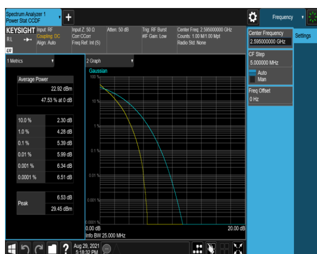
Band41-20MHz-QPSK-40640-100RB#0
