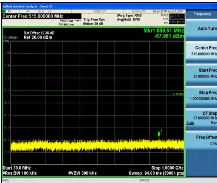
11G-Ant1-2462-30~1000-PASS
