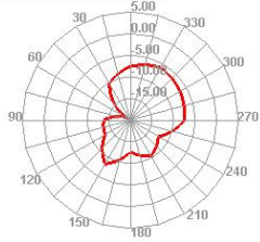
2450.000MHz
