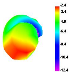
2500.000MHz E1
