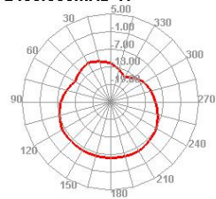
2450.000MHz H
