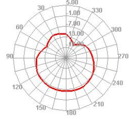
2500.000MHz E2
