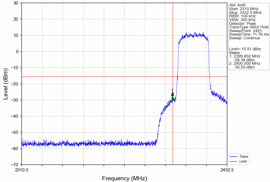
20M_LCH_2412.5MHz_Ant0_NTNV
