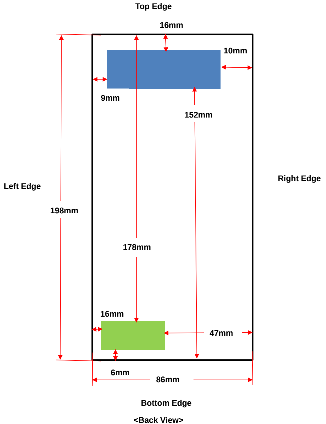
WWAN Antenna
