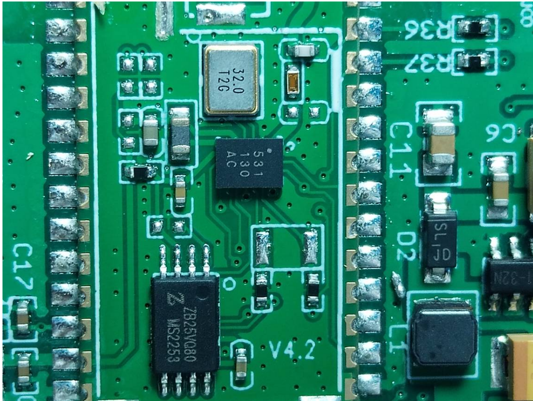
BLE ANT
