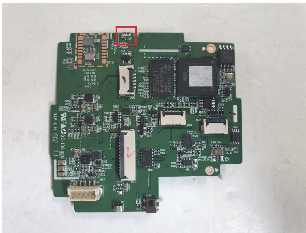
Antenna
