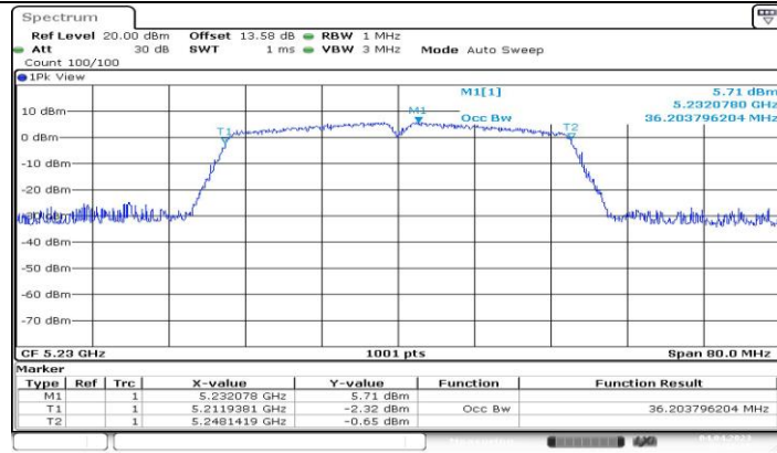
11N40MIMO_Ant0_5230
