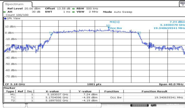
11AX20MIMO_Ant0_5180
