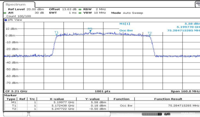
11AC80MIMO_Ant0_5210
