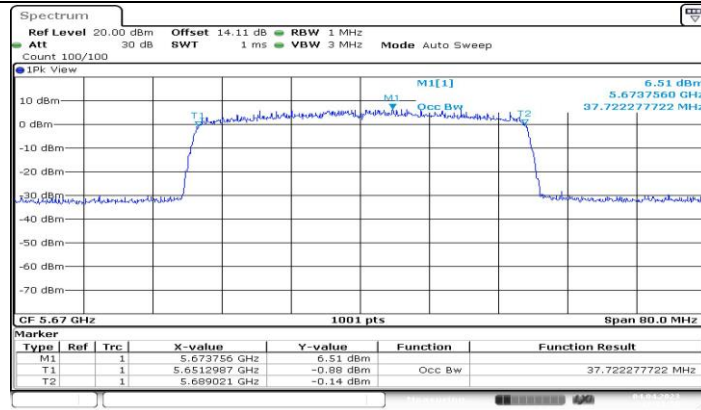
11AX40MIMO_Ant1_5670
