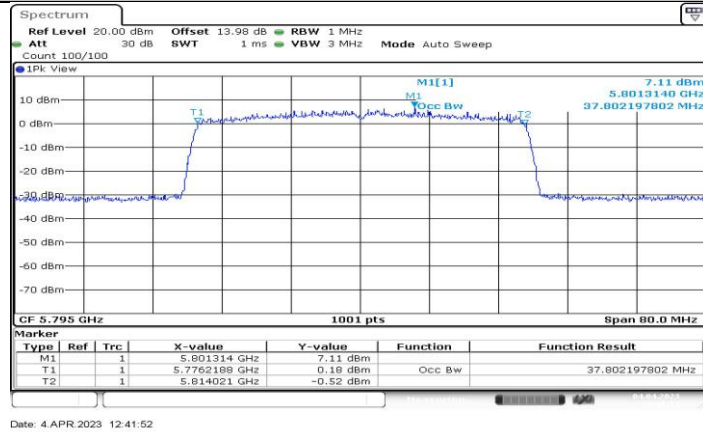
11AX40MIMO_Ant0_5795
