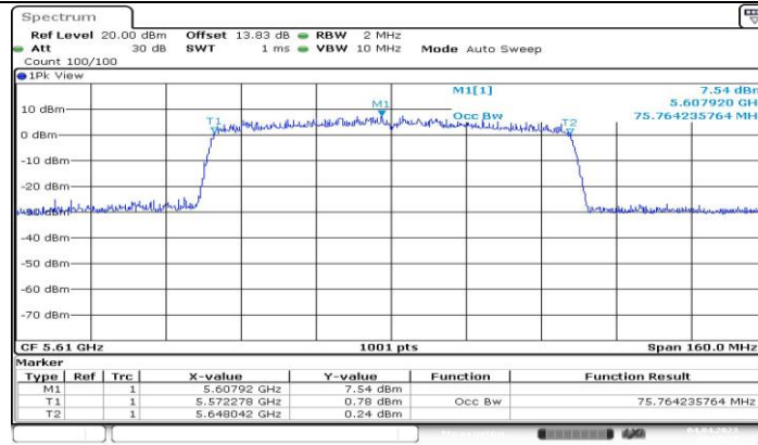
11AC80MIMO_Ant0_5610
