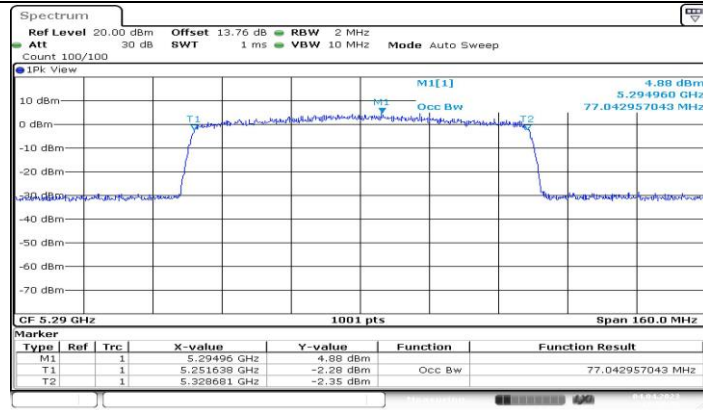
11AX80MIMO_Ant0_5290
